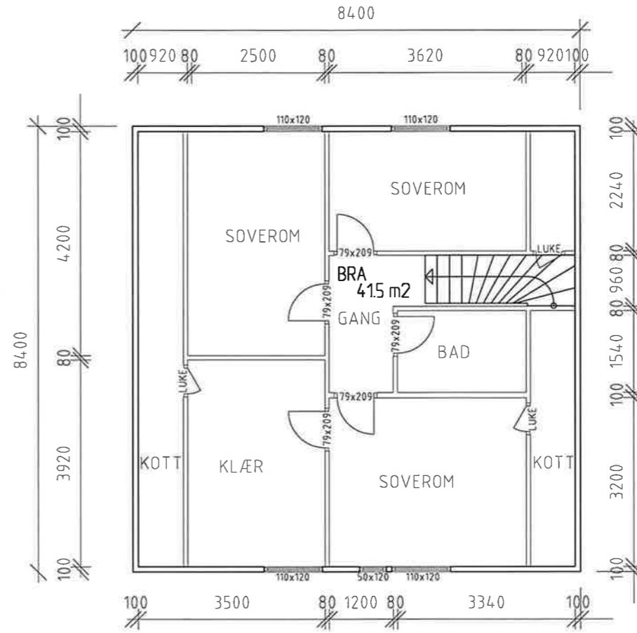
PLAN 2. ETASJE, BTA - 54,8 m 2
