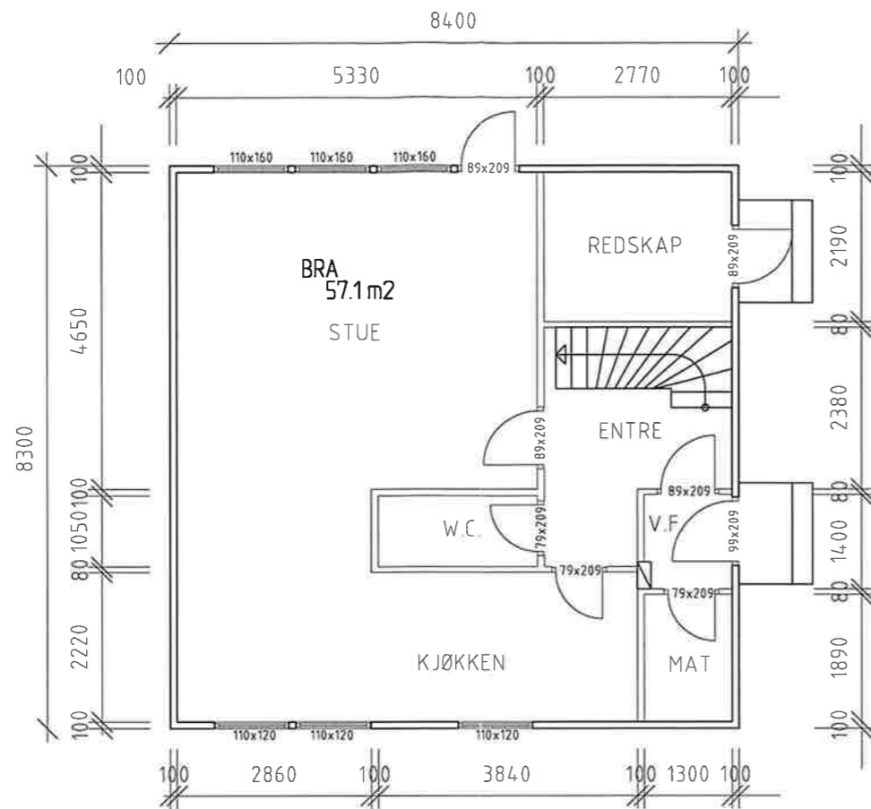
PLAN 1. ETASJE, BTA - 69,7 m 2
