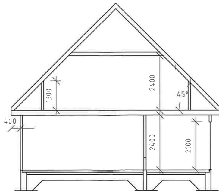
SNITT A-A
